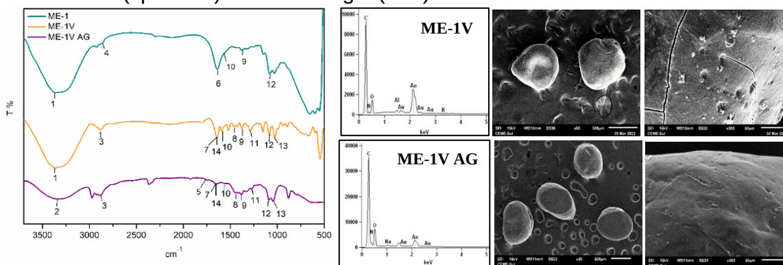
Figura 1 – (A) Espectros FT-IV das micropartículas, sendo Transmitância (%) versus número de onda ( \text{cm}^{-1} ) e (B) Micrografias e espectros de EDS, sendo Intensidade ( \text{cps}\cdot\text{eV}^{-1} ) versus energia (keV).
